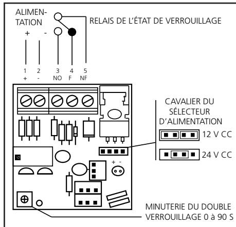
Carte de circuit pour les verrous magnétiques 600 lb
