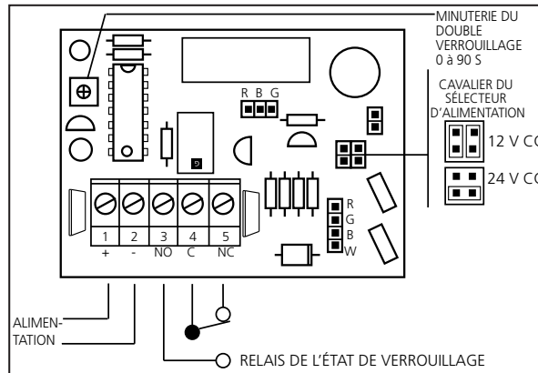
Carte de circuit pour les verrous magnétiques 1 200 lb
